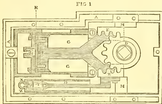
FIG 1. PLAN.
