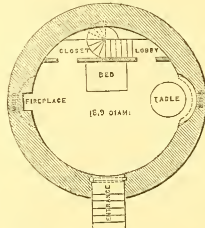
Plan A.
